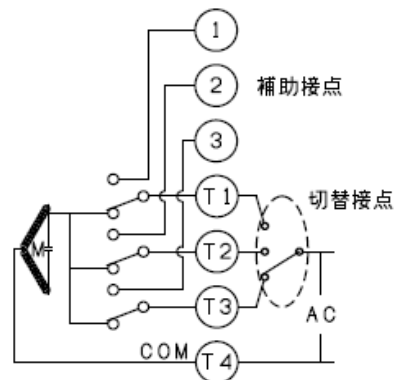
モーター回路図
