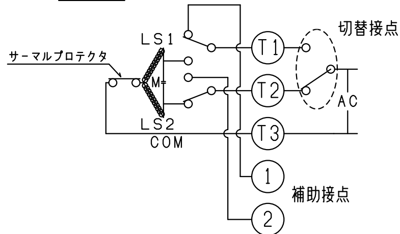
回路図
