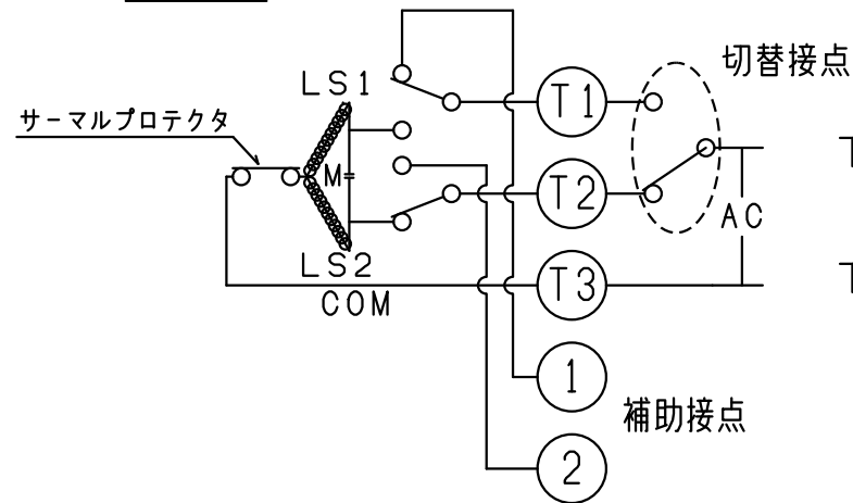
回路図
