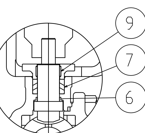
ステム周辺部詳細図
