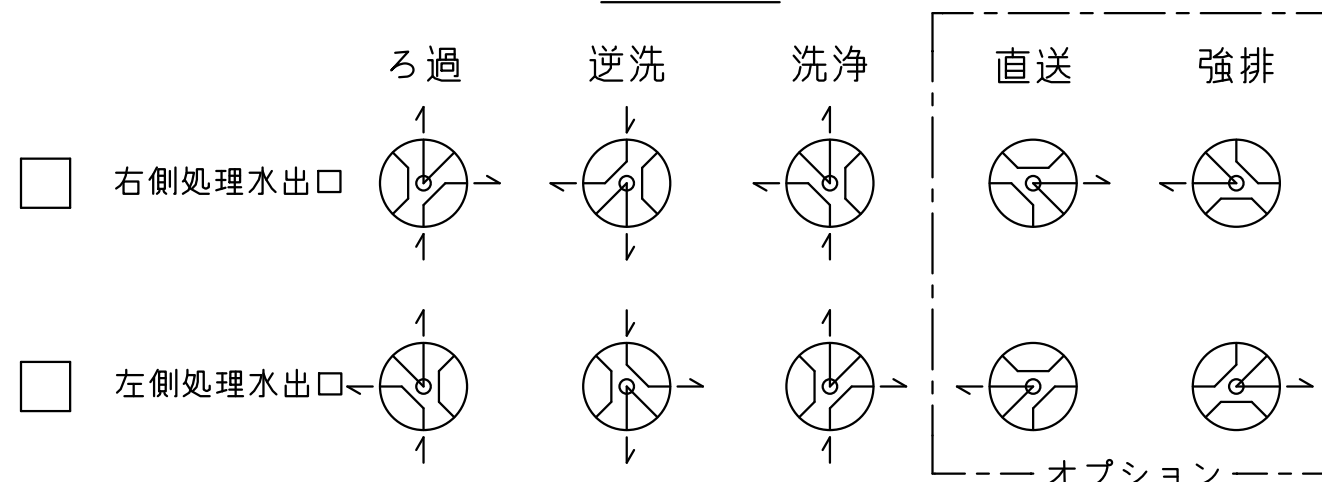
流路説明
