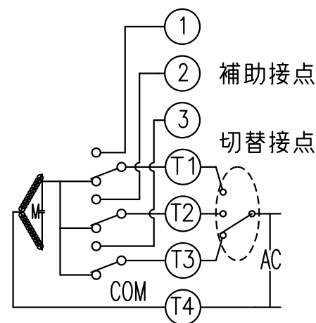
モーター回路図
